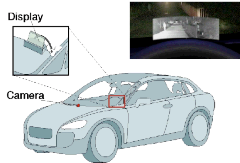
Autoliv NightVision-System im Volvo SCC (Studie)
